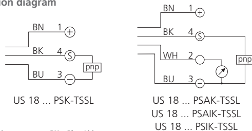
Anschlussschema Connection diagram
