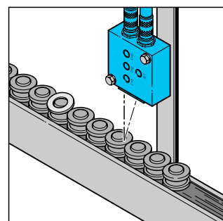
Montageüberwachung, Bolzen montiert Assembly monitoring, bolts fitted
