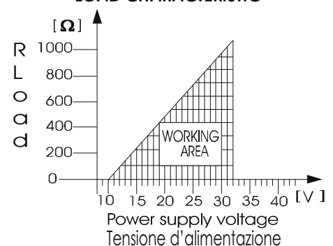
CARATTERISTICA DI CARICO LOAD CHARACTERISTIC
