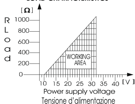
CARATTERISTICA DI CARICO LOAD CHARACTERISTICS
