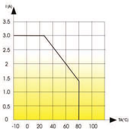
Modello SSR01D/02D/05D-24D Model SSR01D/02D/05D-24D
