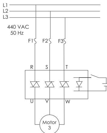
SCHEMI DI COLLEGAMENTO - WIRING DIAGRAMS
