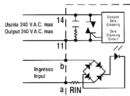
Schema di collegamento carichi in A.C. Wiring diagram A.C. load
