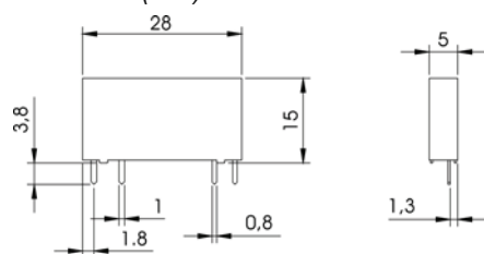
Dimensioni (mm) Dimension (mm)
