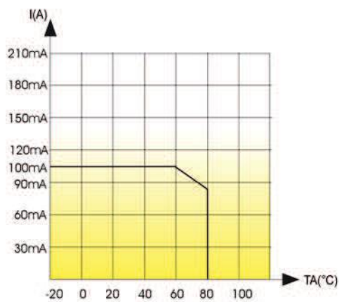
Modello SSR01D/02D/05D-0148 Model SSR01D/02D/05D-0148
